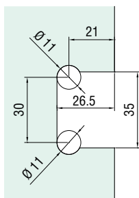
SCHÉMA DE PERÇAGE VANTAIL
