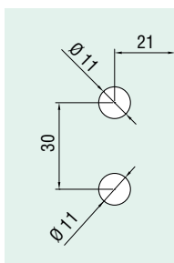
SCHÉMA DE PERÇAGE BORD
